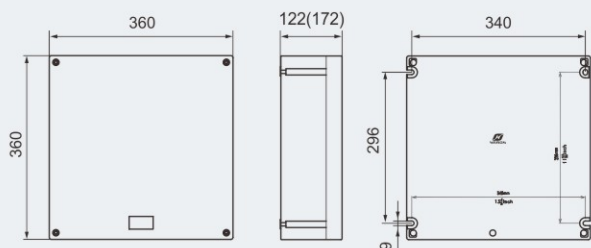
Type V(VB)
