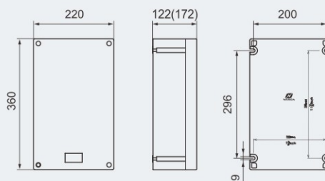
Type IV(IVB)
