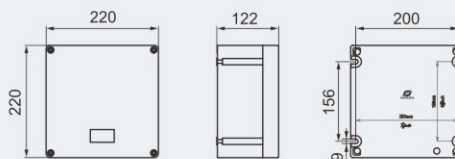
Type VI
